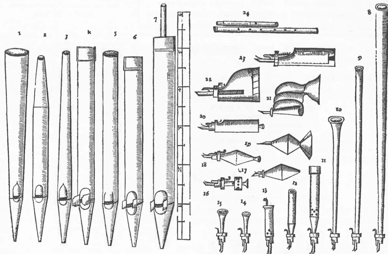
1. Dolcan, 4 ft.; 2. Coppelflöte, 4 ft.; 3. Flachflöte, 4 ft.; 4. Klein Barduen, 8 ft.; 5. Open Flute, 4 ft.; 6. Gedackt, 8 ft.; 7. Rohrlöte or Hohlflöte, 8 ft.; 8. Trompete; 9. Krummhorn, 8 ft.; 10. Schalmei 8, 4 ft.; 11. Sordun, 16 ft.; 12. Zinck: Cornet-discant; 13. Ranckett, 8, 16 ft.; 14. Messing Regale, 8 ft.; 15. Gedempft Regale; 16, 17, 18. Krumbshorn; 19, 20, 21, 22, 23. Various Bärpfeife, 24. Querflöte.
